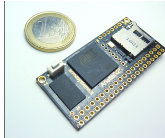
L'Arietta G25 des italiens d'ACME Systems : processeur, mémoire, emplacement micro SD. Le tout sur un adorable petit circuit avec une myriade de GPIO
