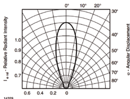
L'angle de diffusion de la led TSAL6200 est très réduit. Ceci est parfaitement adapté pour une télécommande qui est un outil directionnel mais pas nécessairement pour d'autres usages.
