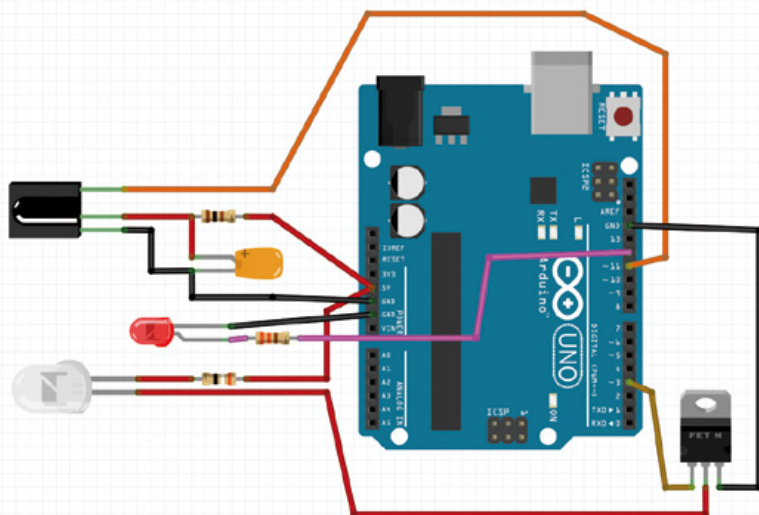
L'angle de diffusion de la led TSAL6200 est très réduit. Ceci est parfaitement adapté pour une télécommande qui est un outil directionnel mais pas nécessairement pour d'autres usages.
