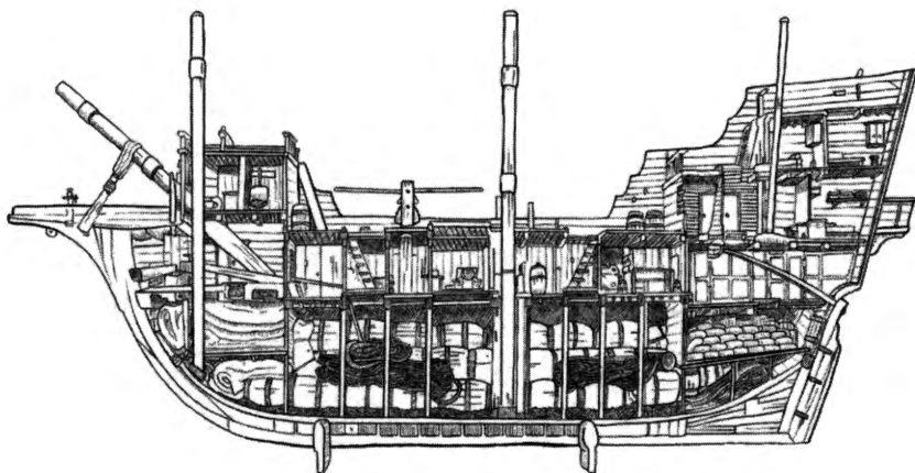
Coupe de la coque d'un galion avec ses trois ponts
